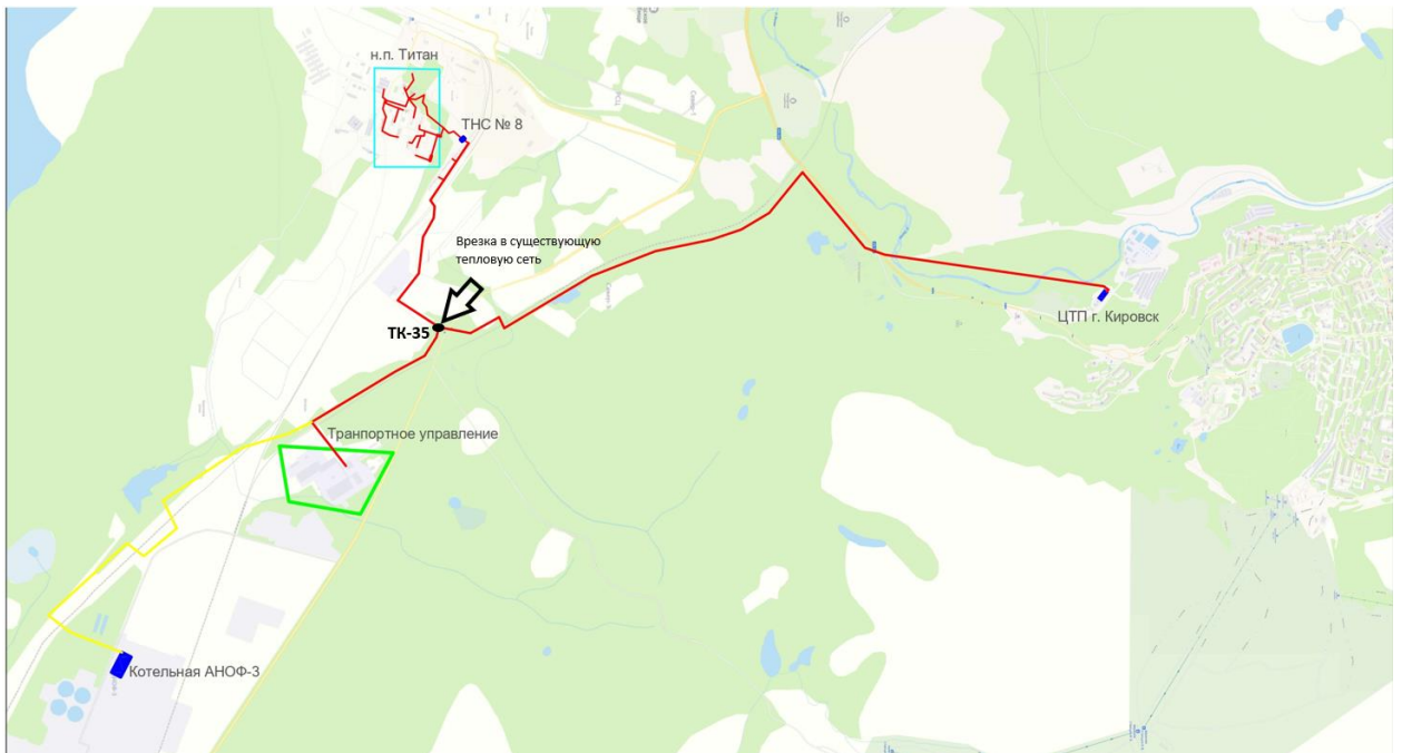
Рисунок 7.9.3 - Предлагаемая схема прокладки тепломагистрали до н.п. Титан
