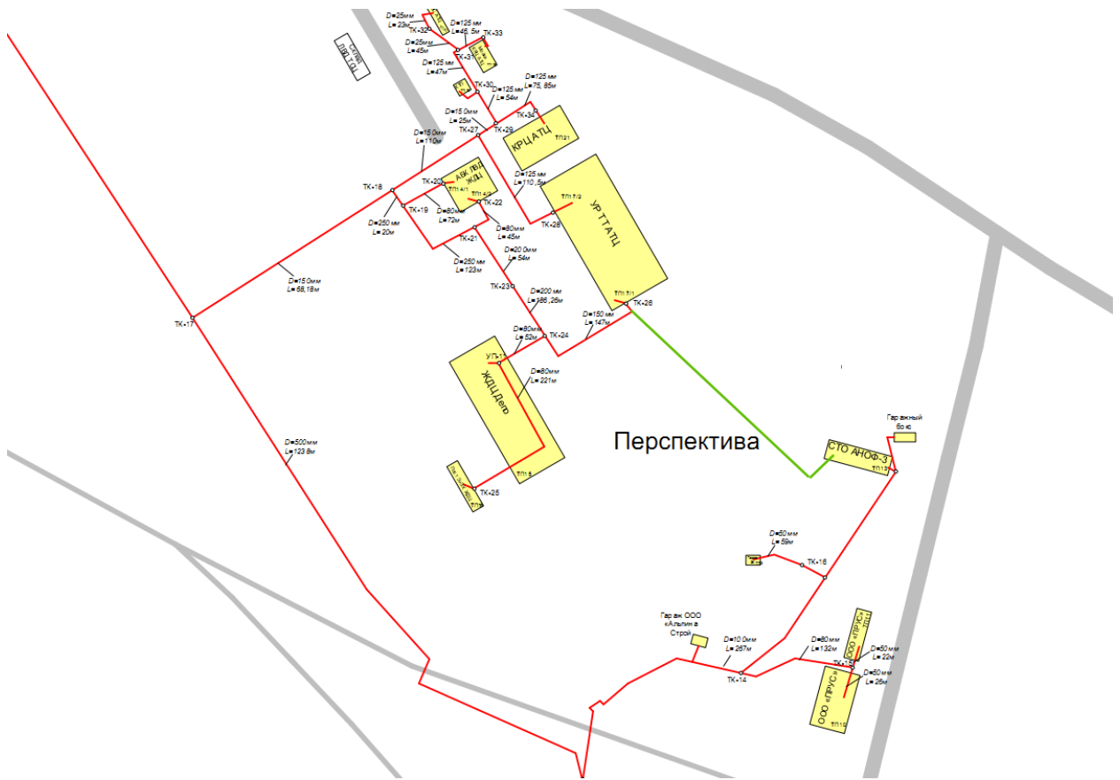
Рисунок 7.9.2 - Перезапитка СТО АНОФ-3 к ТК-26 на территории Транспортного управления КФ АО «Апатит»
