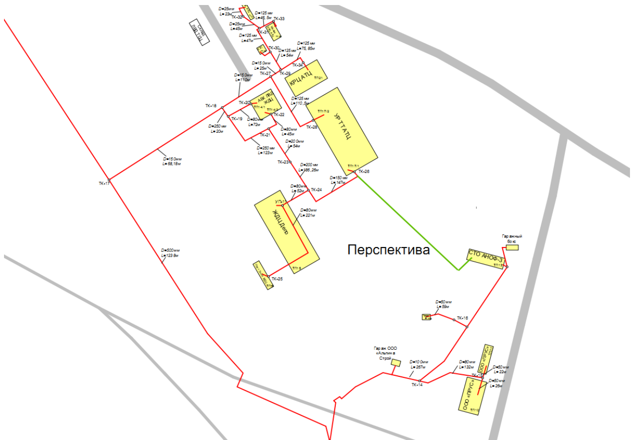
Рисунок 8.5.1 - Перезапитка СТО АНОФ-3 к ТК-26 на территории Транспортного управления КФ АО «Апатит»
