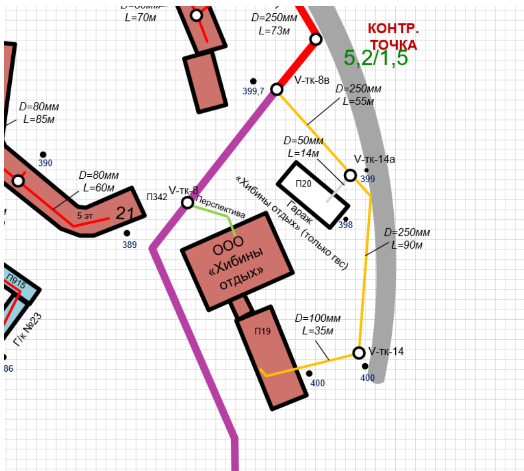
Рисунок 8.7.1 - Ветхий участок тепловой сети от 5-ТК-8в до 5-ТК-14, планируемый к выводу из эксплуатации
