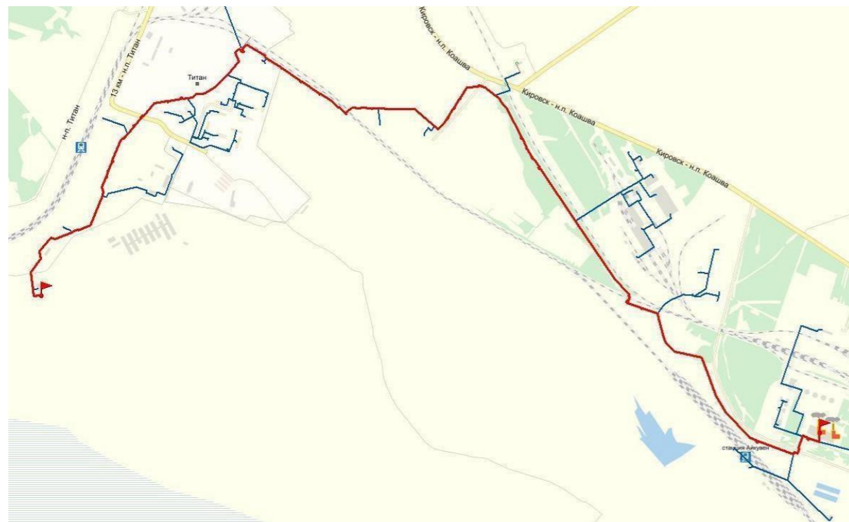
Рисунок 11.4.20 - Направление №3 от котельной АНОФ-3
