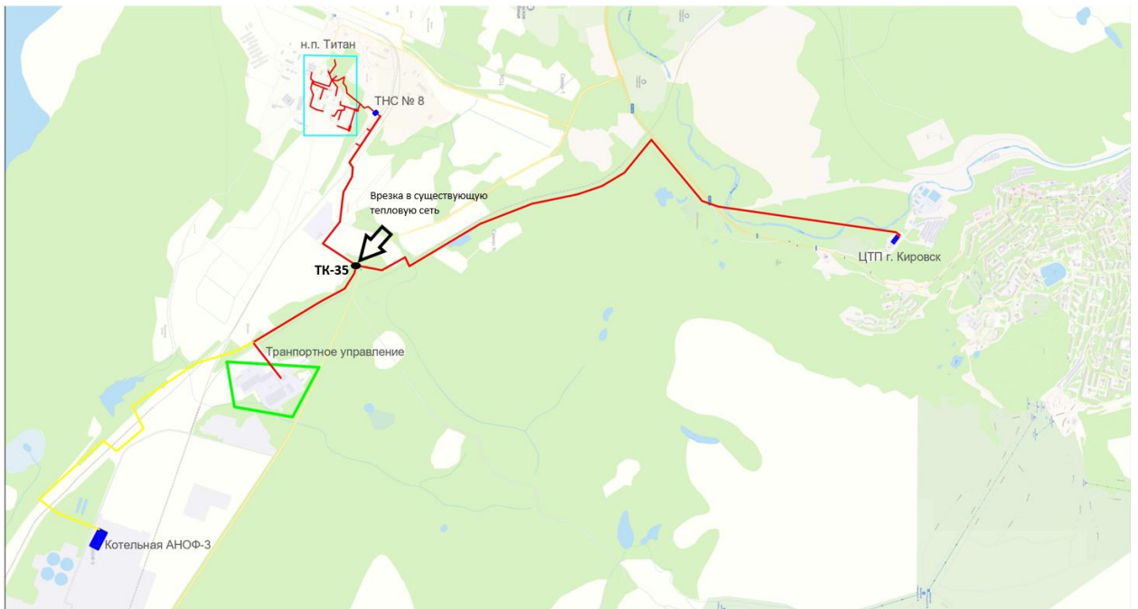
Рисунок 8.5.2 - Предлагаемая схема прокладки тепломагистрали до н.п. Титан
