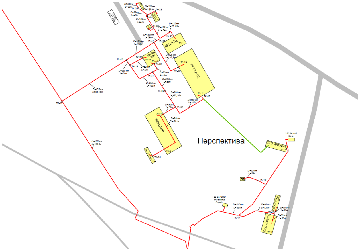
Рисунок 5.1 - Перезапитка СТО АНОФ-3 к ТК-26 на территории Транспортного управления КФ АО «Апатит»
